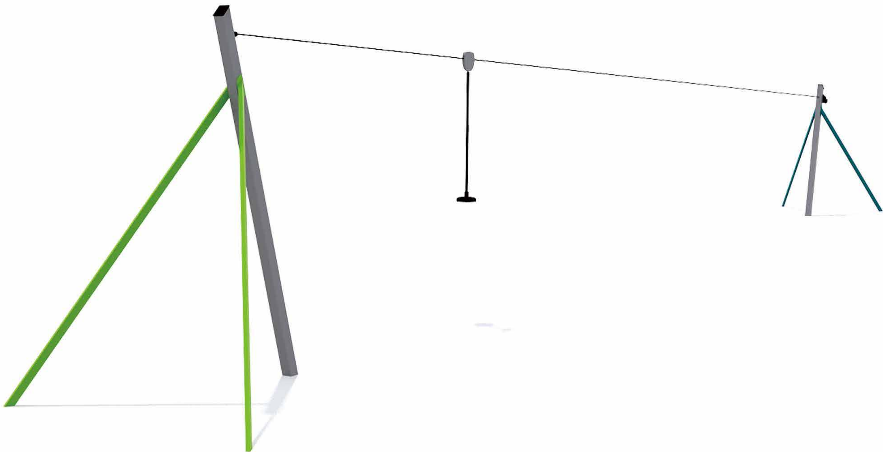
Cód: MC-ZP005 Medidas: 1200 x 250 x 250 cm
